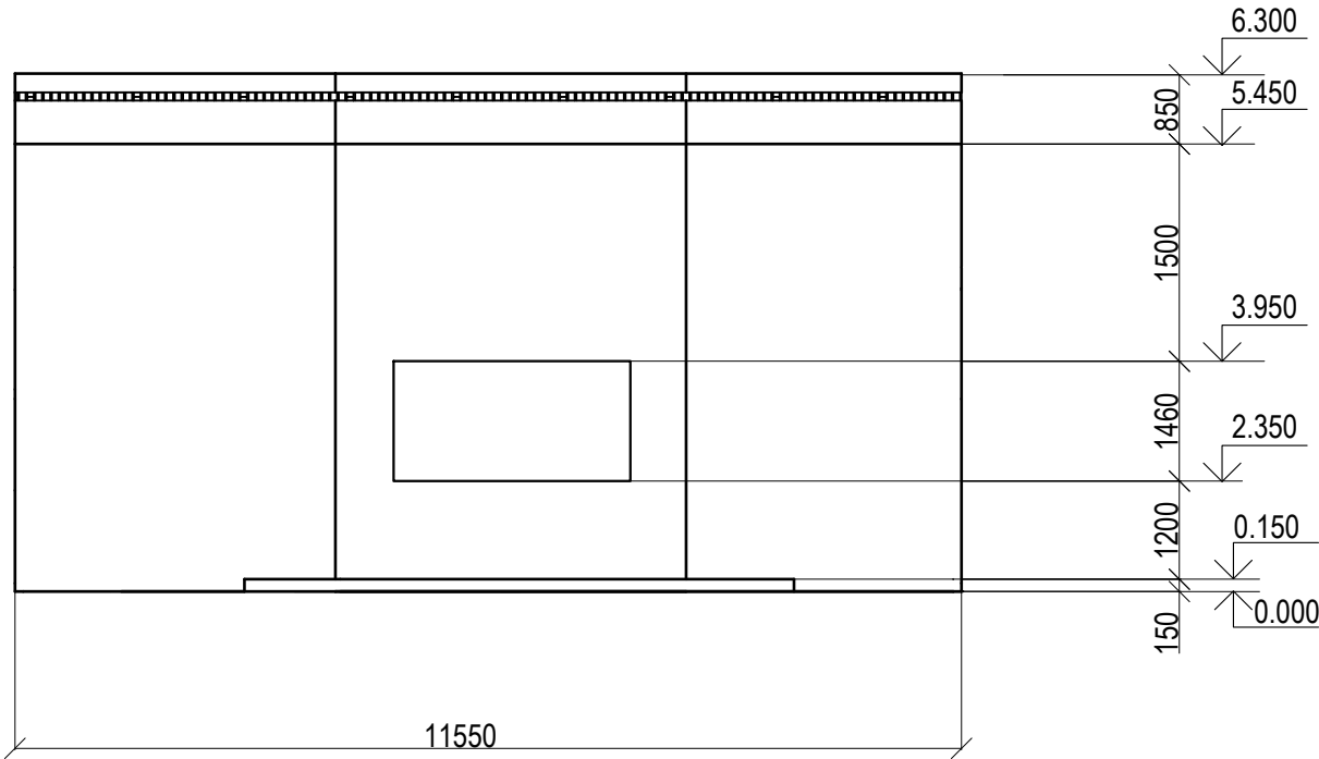
РОЗГОРТКА Б - В
