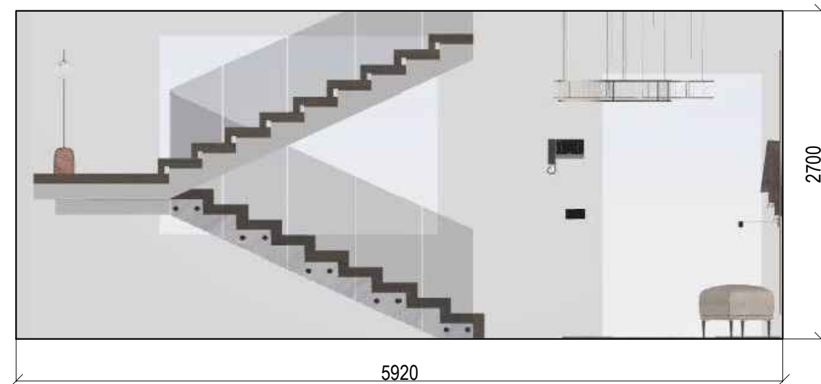
Розгортка 3-1
