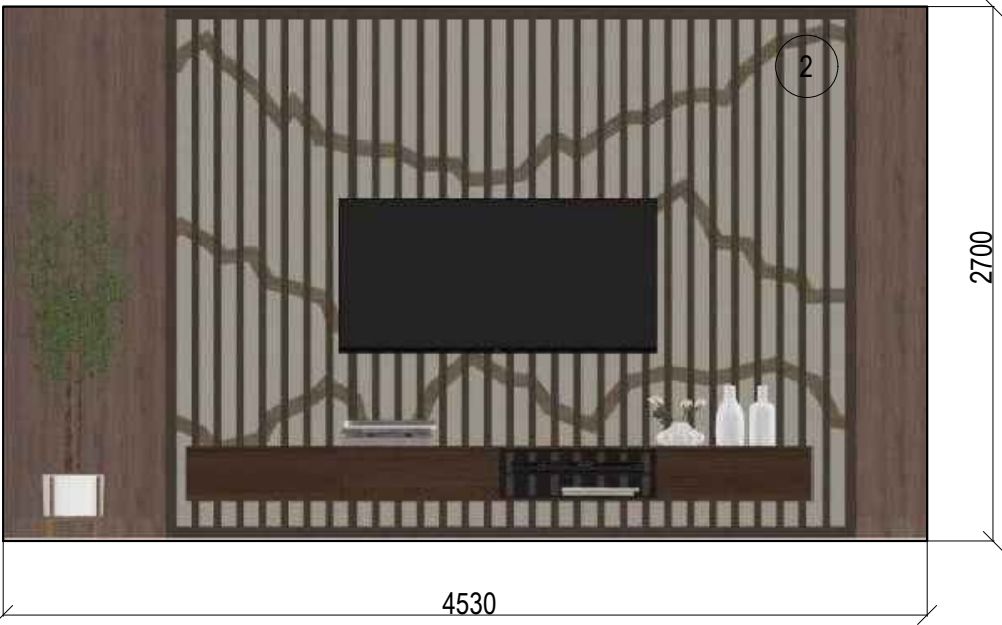
Розгортка 12-13
