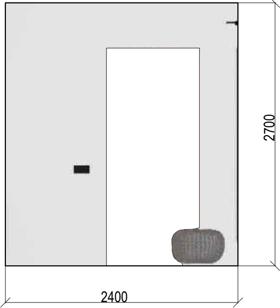
Розгортка 23-18
