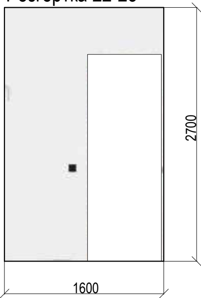
Розгортка 22-23
