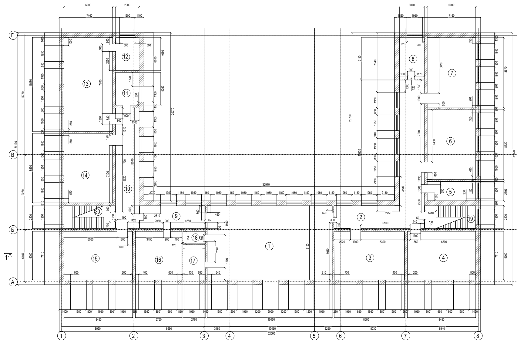
Експлікація приміщень
