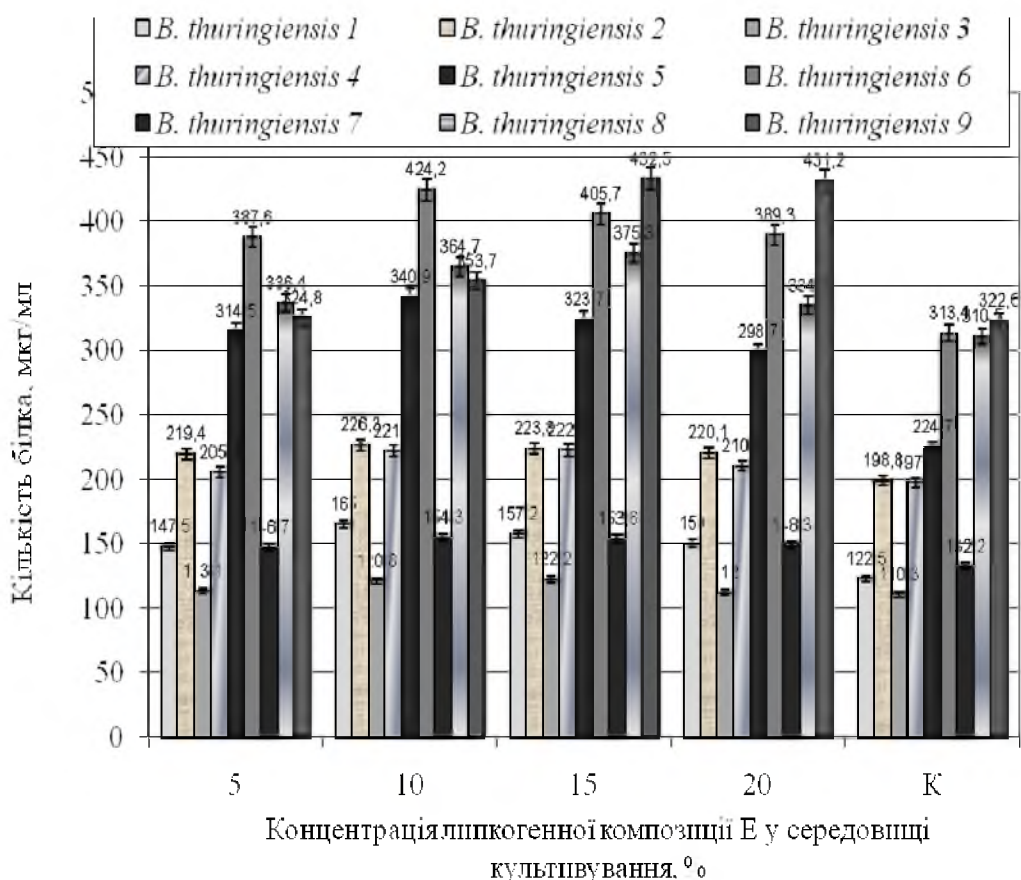
Рис. 2. Синтез білка ізолюваними штамами Bacillus thuringiensis за присутності в поживному середовищі липкогенної композиції Е.
