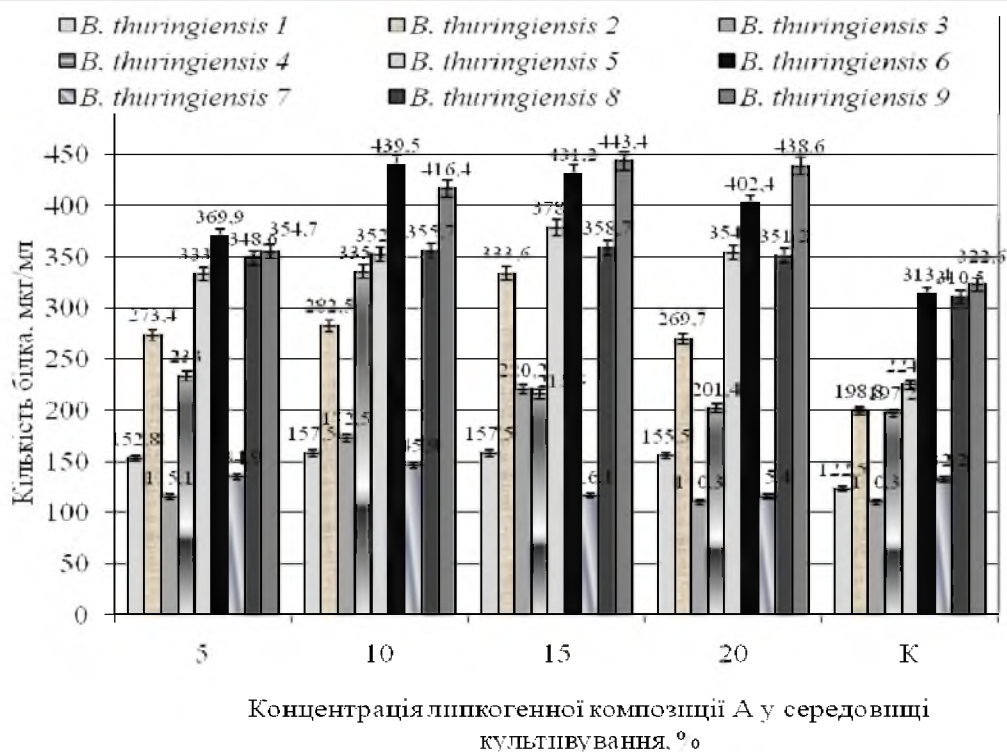
Рис. 1. Синтез білка ізолюваними штамами Bacillus thuringiensis за присутності в поживному середовищі липкогенної композиції А.
