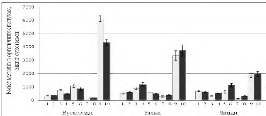
Рис. 2. Вміст металів в органічних сполуках клітин Ch. vulgaris : 1, 2 – \text{Se}^{4+} + \text{Co}^{2+} (контроль, дослід); 3, 4 – \text{Se}^{4+} + \text{Mn}^{2+} (контроль, дослід); 5, 6 – \text{Se}^{4+} + \text{Cu}^{2+} (контроль, дослід); 7, 8 – \text{Se}^{4+} + \text{Zn}^{2+} (контроль, дослід); 9, 10 – \text{Se}^{4+} + \text{Fe}^{3+} (контроль, дослід).
