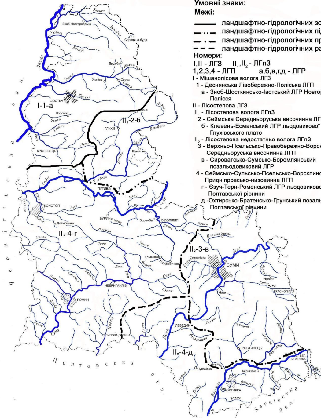
Рис. 1. Ландшафтно-гідрологічне районування території Сумської області
