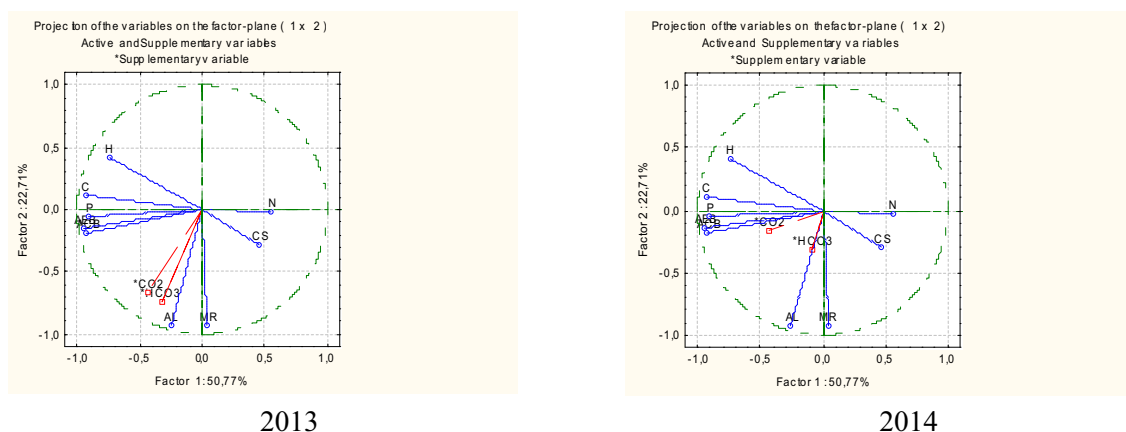
Рис. 2. Діаграми проєкцій змінних показників на факторну-площину 1-2
