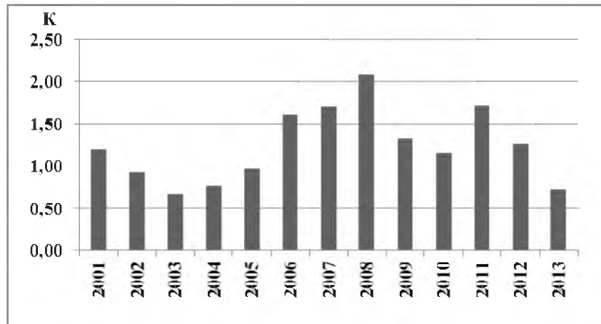
Рис. 2. Зміна коефіцієнту зовнішнього водообміну (K) водосховища Сасик з 2001 по 2013 р.
