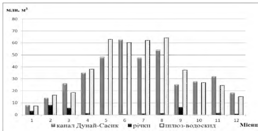
Рис. 1. Внутрішньорічний розподіл деяких складових водного балансу водосховища Сасик (2001- 2013 рр.)
